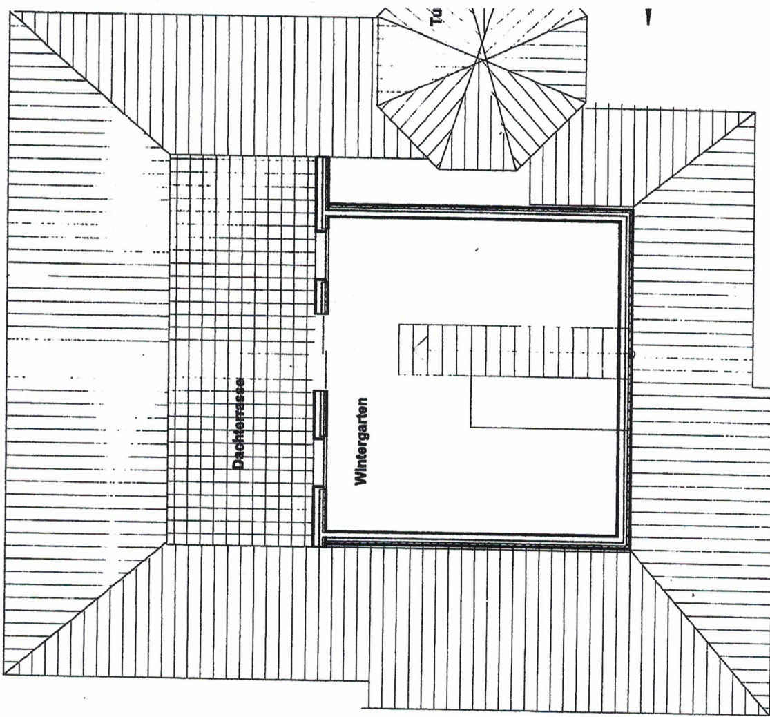
Dachgeschoss
